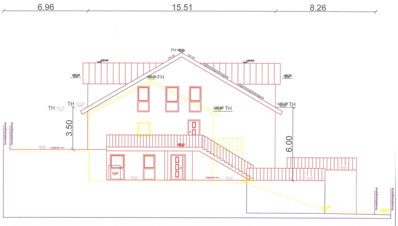
Ansicht West
