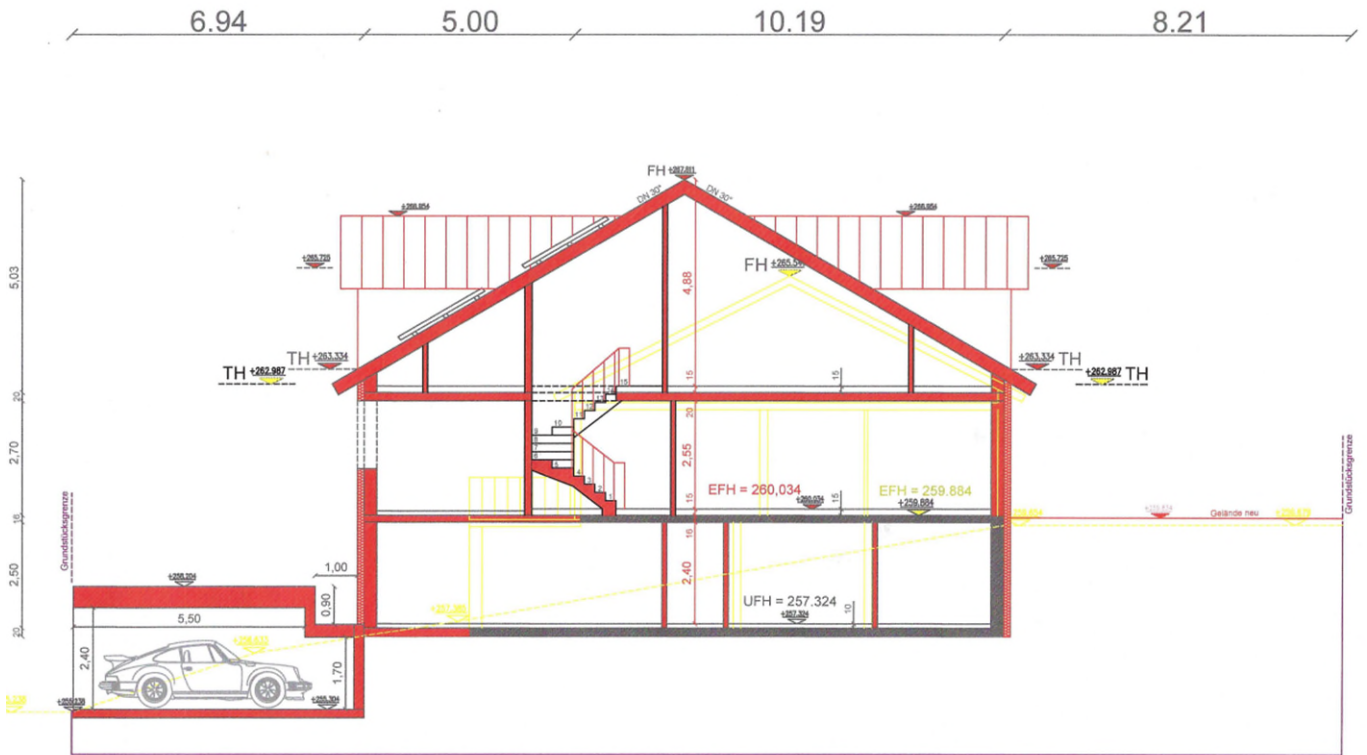
Schnitt A-A
